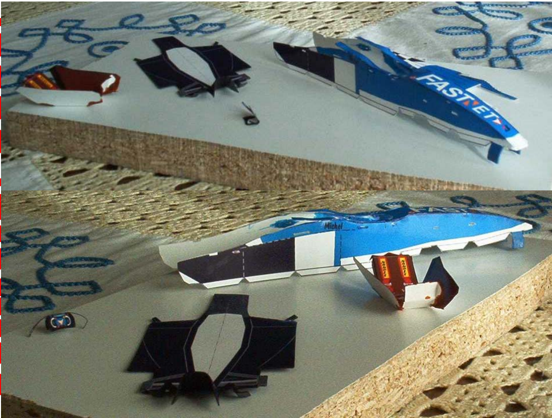
Fase 2: sospensioni, aircscope, deflettori, fiancate e cassoni dei radiatori laterali.
